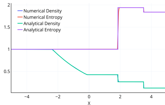
Рис. 2. Профиль плотности и энтропии ( P/\rho^\gamma , \gamma - показатель адиабаты) при решении задачи Сода и их аналитическое решение.
