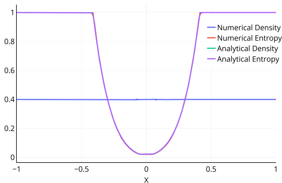
Рис. 1. Профиль плотности и энтропии ( P/\rho^\gamma , \gamma - показатель адиабаты) при решении задачи Эйфельдта
