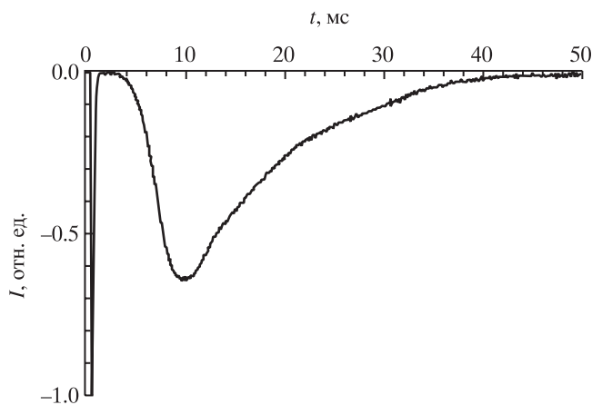
Рис. 5. Сигнал с коллимированного фотоэлектронного умножителя, зарегистрированный на расстоянии y = 20 мм от поверхности антенны при автовоспламенении керосина в воздухе в условиях поверхностного СВЧ-разряда при \tau = 100 мкс, W = 55 кВт, p = 760 Тор.
