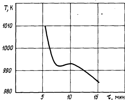
Рис. 2. Термограмма кристаллизации бария
