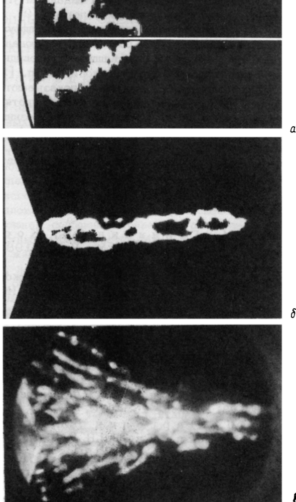
Рис. 2. Термограммы распределения интенсивности излучения на входе (а) и выходе (б) СВЧ-аксикона. Структура СВЧ разряда в поле аксикона при давлении воздуха 3 Тор (в).
