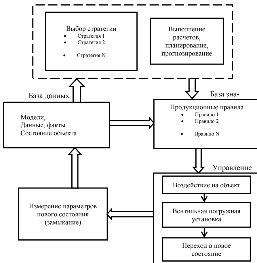
Рис. 2. Схема интеллектуального анализа и управления
