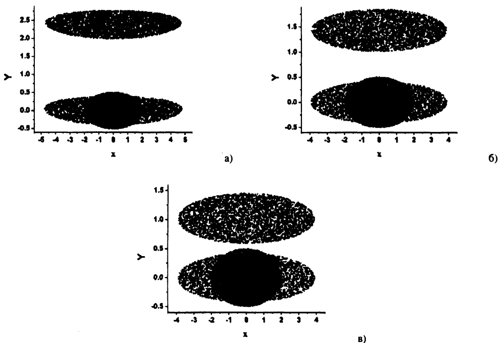
Рис.6. Распределения частиц в анализирующей плоскости.
