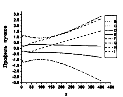
Рис.7. Профили пучков и распределения плотности частиц на входе сепаратора и в плоскости анализирующей щели.
