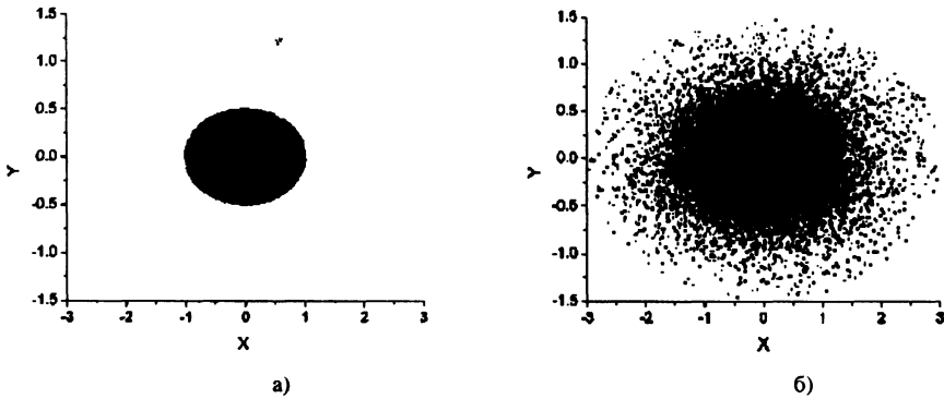
Рис.1. Начальные распределения частиц
