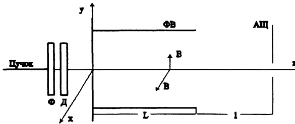
Рис.2. Схема сепаратора Вина, принятая в рассматриваемой модели: Ф – фокусирующая линза, Д – дефокусирующая линза, ФВ – фильтр Вина, АЩ – анализирующая щель
