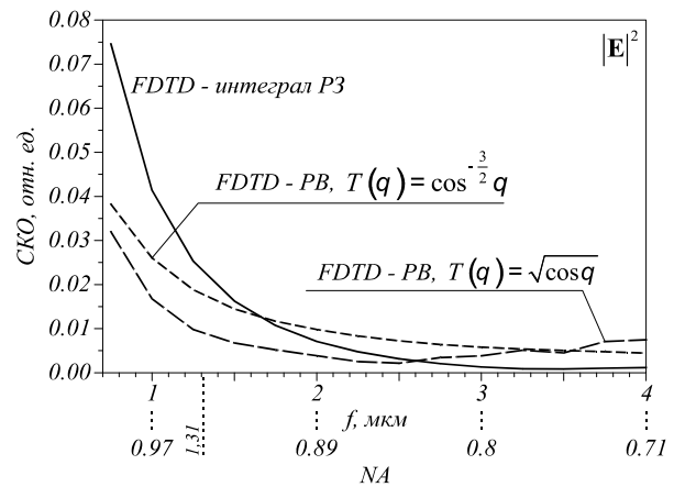
Рис. 6. Зависимость СКО между интенсивностями, полученными с помощью FDTD-метода и преобразования Ричардса–Вольфа, интеграла Рэлея–Зоммерфельда от фокусного расстояния f . Падающее поле – Гауссов пучок с радиусом w = 3 мкм с круговой поляризацией, ограниченный апертурой R = 4 мкм
