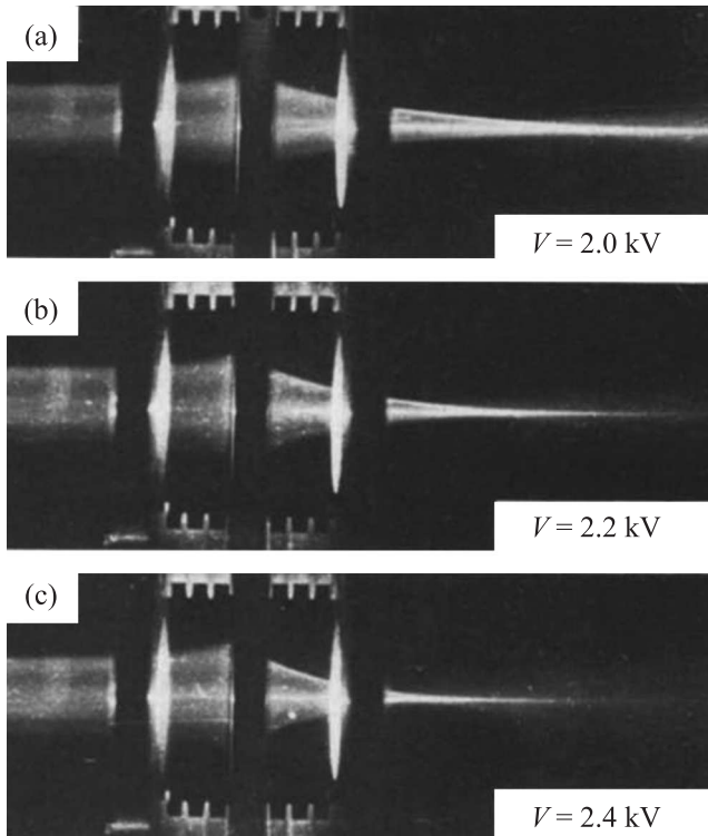
Рис. 3. Снимок светящегося пучка однозарядных ионов диспрозия, проходящего через одиночную электростатическую линзу при различных значениях потенциала V , приложенного к ее среднему электроду. Энергия ионов E_0 = 3 кэВ, ток ионного пучка I_0 = 8 \cdot 10^{-6} А. Диаметр пучка на входе в линзу \sim 18 мм. Диаметр отверстий в электродах линзы 24 мм
