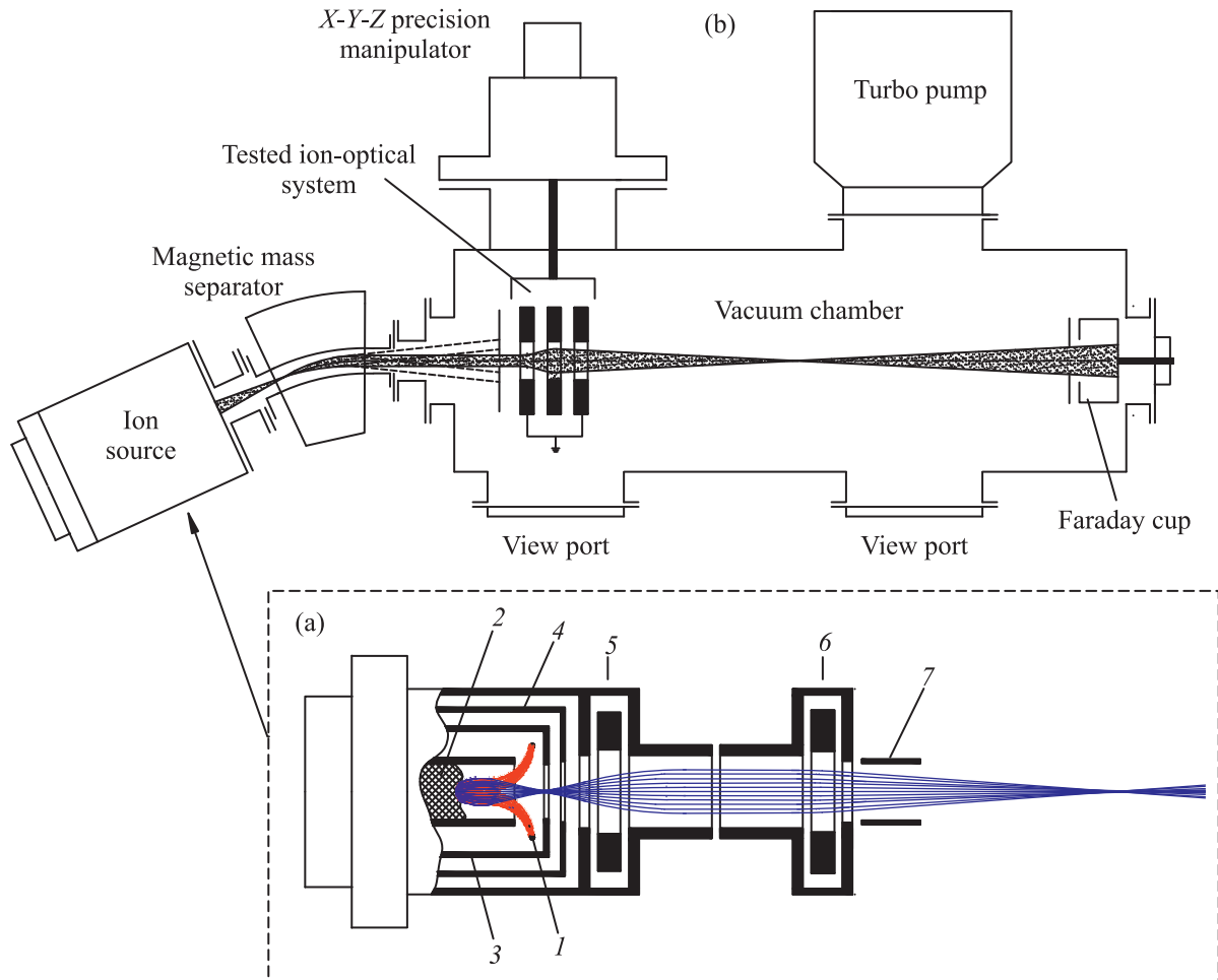
Рис. 1. (Цветной онлайн) (а) – Схема источника ионов: 1 – катод, 2 – резервуар (анод) для загрузки рабочего вещества, 3 – отражающий электрод, 4 – ускоряющий электрод, 5 и 6 – одиночные электростатические линзы, 7 – дефлектор. На рисунке приведены траектории электронного и ионного пучков. (б) – Схема экспериментального прибора для исследования “светящихся ионных пучков”
