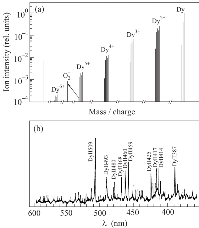
Рис. 2. (а) – Диаграмма масс-спектра пучка ионов Dy^{q+} ( q = 1 \div 6 ). Для каждого значения q сигнал содержит пять пиков, соответствующих стабильным изотопам с массами 160, 161, 162, 163 и 164. (б) – Оптический спектр свечения пучка возбужденных однозарядных ионов диспрозия, измеренный для ионного пучка с энергией ионов E_0 = 3 кэВ и током пучка I_0 = 2 \cdot 10^{-6} А
