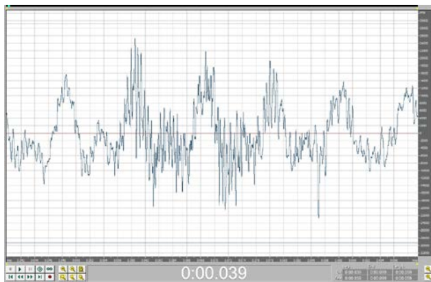
Рис. 11. Общая длительность 0,059 секунды. Область максимума нелинейных искажений. Вначале высокая скорость нарастания, затем, переход на более гармоничные колебания.
