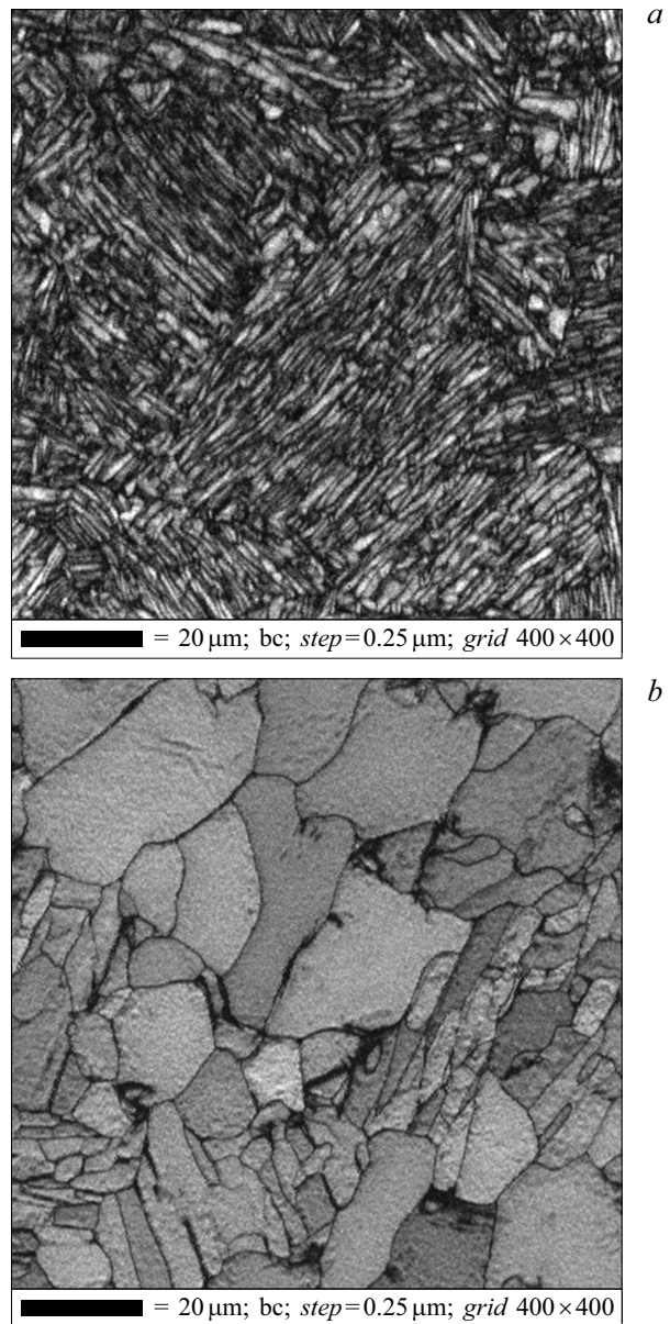
Рис. 5. EBSD-карты качества (band contrast) образцов СЛС-титана VT1-0 в исходном состоянии (а) и после отжига при 800°C (б).
