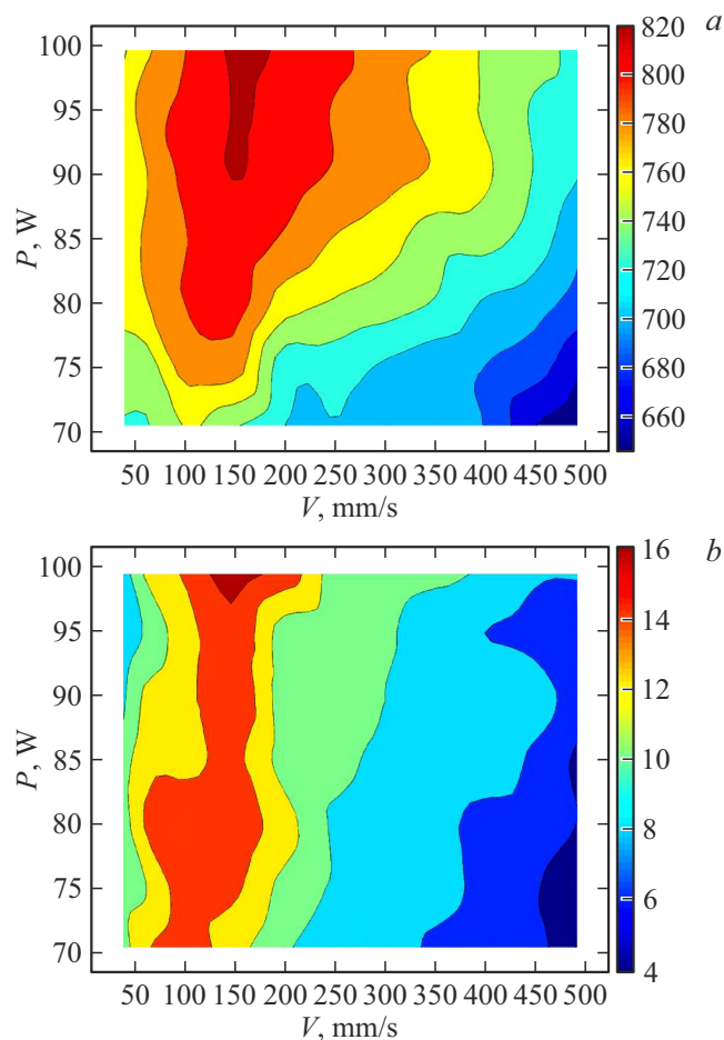
Рис. 2. Зависимость предела прочности ( a ) и удлинения после разрыва ( b ) СЛС-титана VT1-0 от мощности излучения P и скорости сканирования V .
