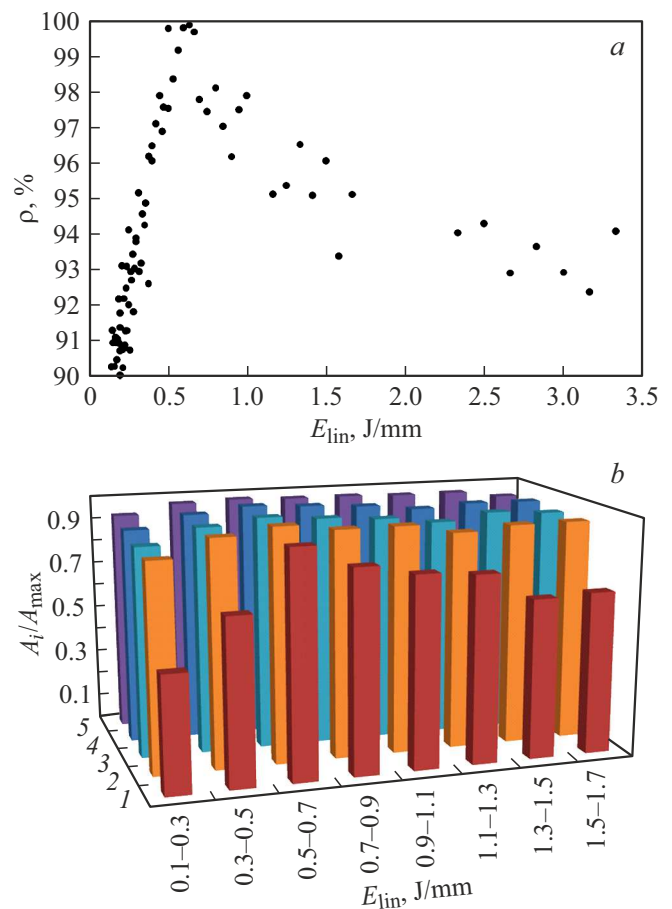
Рис. 6. Зависимость физико-механических характеристик титана VT1-0 от линейной плотности энергии E_{lin} при СЛС: а — зависимость для относительной плотности \rho ; б — диаграмма для нормированных значений характеристик A_i/A_{max} : 1 — удлинение после разрыва, 2 — предел текучести, 3 — предел прочности, 4 — относительная плотность, 5 — модуль Юнга.
