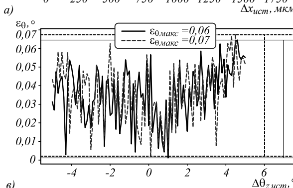
Рис. 16. Абсолютные погрешности определения смещений между волоконной линзой и торцом ФИС: погрешности определения продольного смещения при угловом смещении 1° (а); максимальные погрешности определения продольного смещения в зависимости от угла волоконной линзы (б); погрешности определения углового смещения на расстоянии 600 мкм (в); максимальные погрешности определения углового смещения в зависимости от расстояния (г); на графиках: сплошная линия – прямой ход, пунктирная – обратный ход
