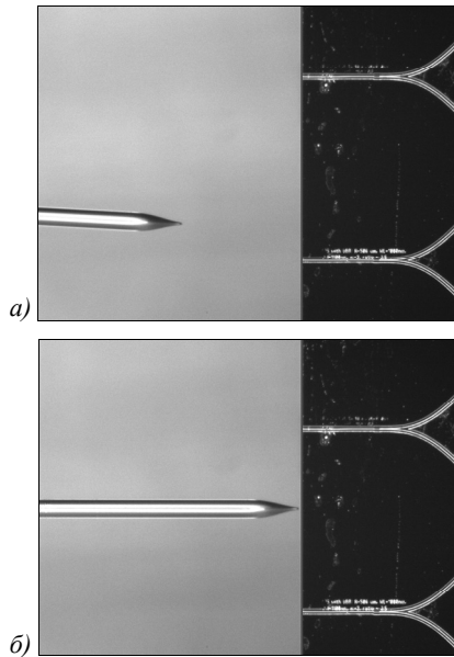
Рис. 3. Изображения области юстировки волоконной линзы и фотонной интегральной схемы: до первичной юстировки (а); после первичной юстировки (б)
