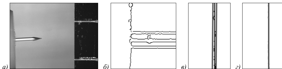
Рис. 9. Поиск границы ФИС: исходное изображение (а); увеличенный фрагмент изображения вблизи волновода с выделенными границами (б); прямые, найденные с помощью преобразования Хафа и отобранные по критерию (б) (в); искомая прямая (г)
