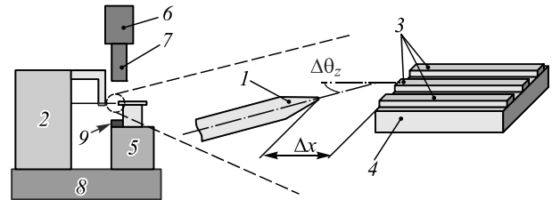
Рис. 4. Система технического зрения: 1 – волоконная линза; 2 – платформа; 3 – каналные волноводы; 4 – фотонная интегральная схема; 5 – столик; 6 – камера; 7 – телецентрический объектив; 8 – виброизолирующее основание; 9 – источник освещения (проходящий свет)
