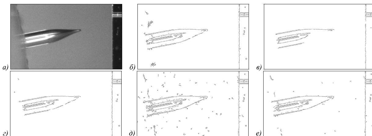
Рис. 7. Выделение границ методом Кэнни: фрагмент исходного изображения (а); результаты при различных значениях нижнего и верхнего порогов (б–е): 20:80 (б), 40:120 (в), 44:89 (г), 31:62(д), 35:71 (е); пороги заданы вручную (б, в), пороги рассчитаны упрощенным способом (г), пороги рассчитаны по формулам (3) при разбиении изображения на 4 и 9 частей соответственно (д, е)
