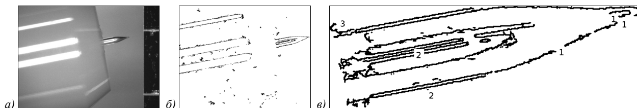
Рис. 10. Поиск контуров: исходное изображение (а), фрагмент левой части изображения с выделенными границами (б), увеличенный фрагмент изображения контуров волоконной линзы: 1 – ложные разрывы, 2 – дублирование линий, 3 – бахрома (в)
