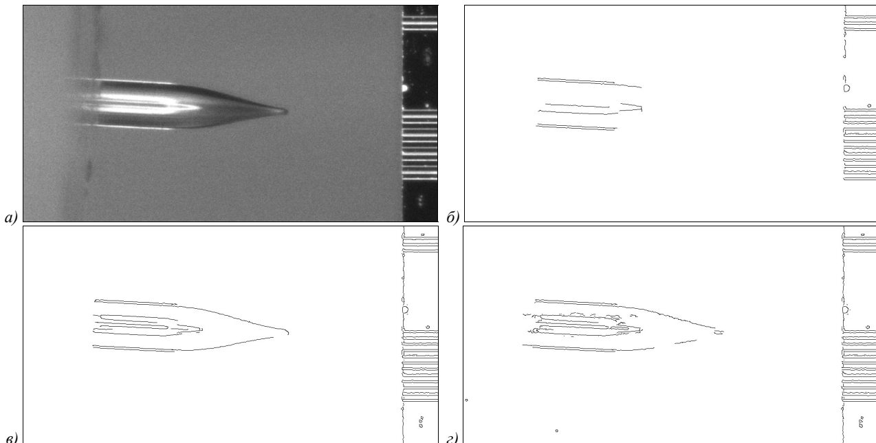
Рис. 8. Выделение границ в сложном случае с помощью детектора Кэнни: фрагмент исходного изображения (а); адаптивные пороги 89:179 (б); предварительная фильтрация шумов, адаптивные заниженные пороги 45:90 (в); ручные пороги 45:90 (без предварительной фильтрации шумов)(г)
