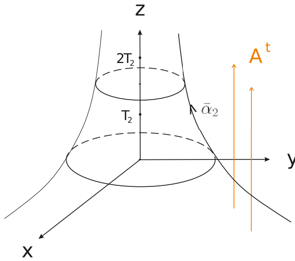
Рис. 4.1. Прообраз \bar{\alpha}_2 образующей \alpha_2 полнотория \mathbb{V}_2 Fig 4.1. Preimage of \bar{\alpha}_2 of generator \alpha_2 of solid torus \mathbb{V}_2
