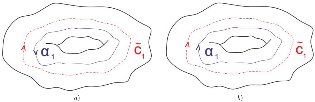
Рис. 4.2. а) несогласованная ориентация циклов c_1 и c_2 ; б) согласованная ориентация циклов c_1 и c_2
