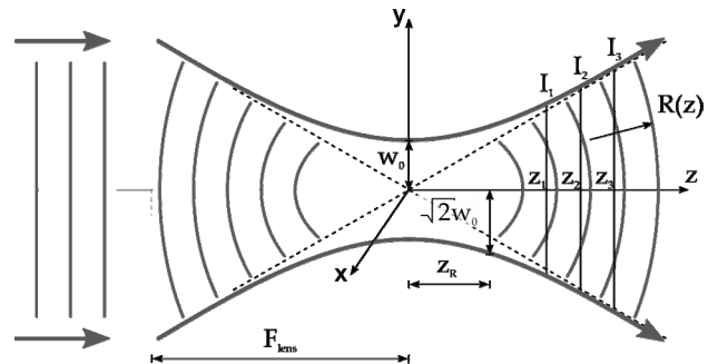
Рис. 1. Пространственная структура лазерного пучка
