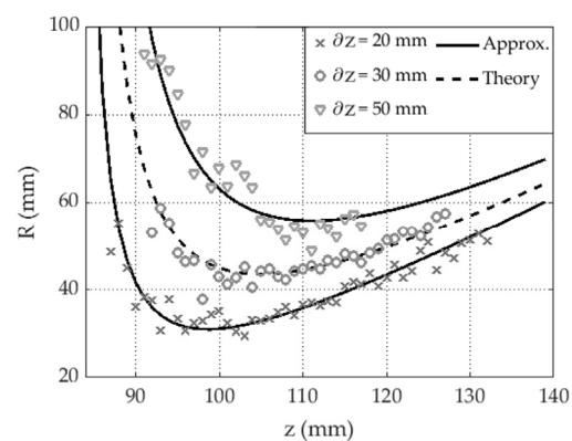
Рис. 5. Зависимость радиуса кривизны R(z_2) от продольной координаты для нескольких \Delta z
