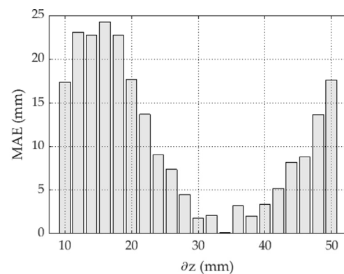
Рис. 6. Зависимость средней абсолютной ошибки от величины \Delta z
