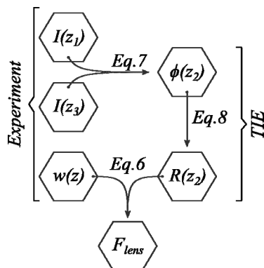
Рис. 2. Алгоритм расчета параметров линзы
