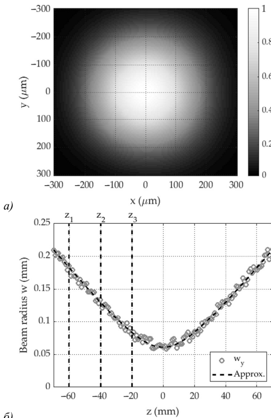
Рис. 4. (а) Поперечное распределение интенсивности пучка, (б) продольное сечение распределения интенсивности
