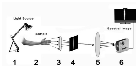
Рис. 2. Оптическая схема эксперимента: 1 – источник освещения, 2 – объект, 3 – линза, 4 – целевая диафрагма, 5 – СДЛ, 6 – камера Basler acA 1920-40um
