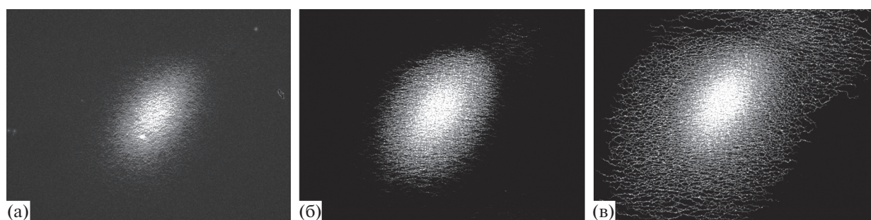
Рис. 5. Изображения поврежденной свинцовой пленки при воздействии на нее разным количеством ТГц-импульсов: (а) – 1 импульс, (б) – 5, (в) – 600, с напряженностью электрического поля 23 МВ/см.
