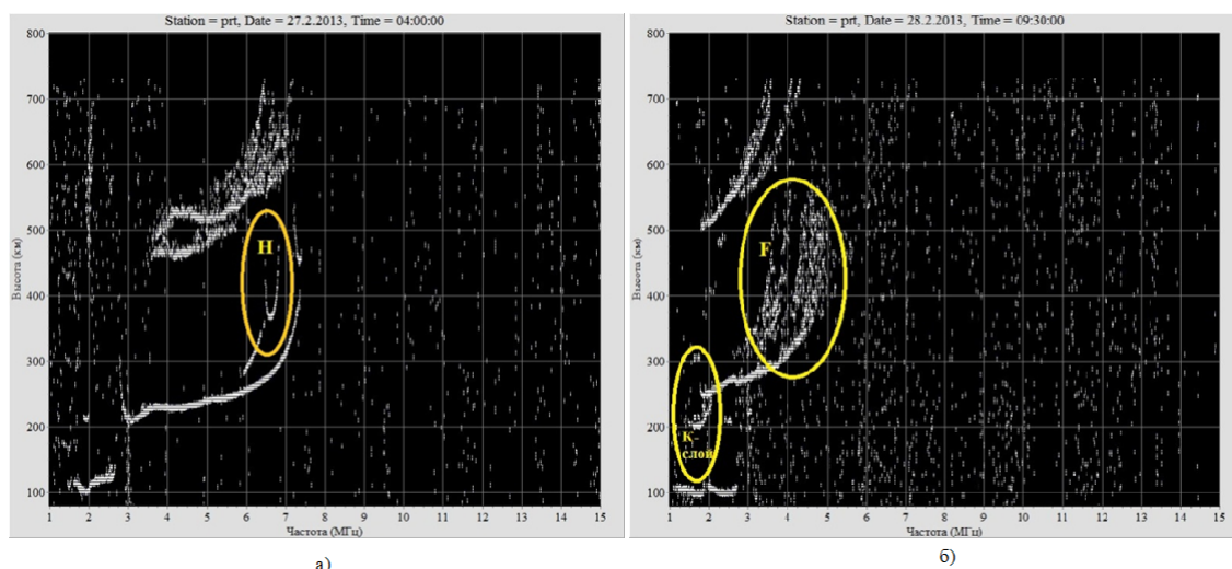
Рис. 2. Примеры аномального поведения параметров ионосферы. а) - расслоение слоя F2 по частоте и высоте (режим "H" перемещающиеся ионосферные возмущения). б) - на фоне спокойной магнитосферы формирование за 1-3 дня диффузионного слоя F2 ( F2 -spread) длительностью в несколько часов (режим "F"); формирование K -слоя, за счет высыпания заряженных частиц из радиационных поясов
