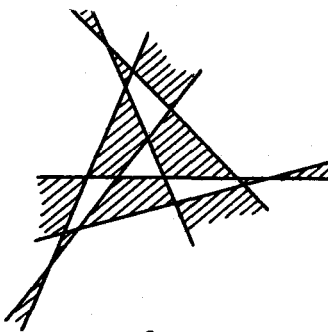
Рис. 2. Четыре возможных комбинаторных типа конфигураций шести прямых общего положения. Закрашенная область представляет W^- .
