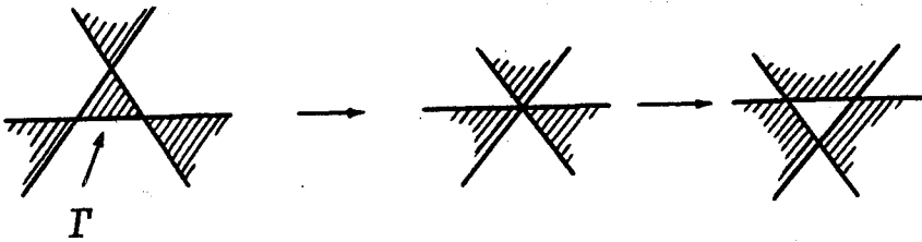
Рис. 4. Элементарное преобразование конфигурации: стягивание треугольника \Gamma сопровождается сдутием накрывающего цикла \tilde{\Gamma} \subset Y^\epsilon .
