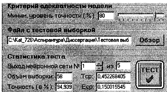
Рис. 7. Пример тестирования полученной модели
