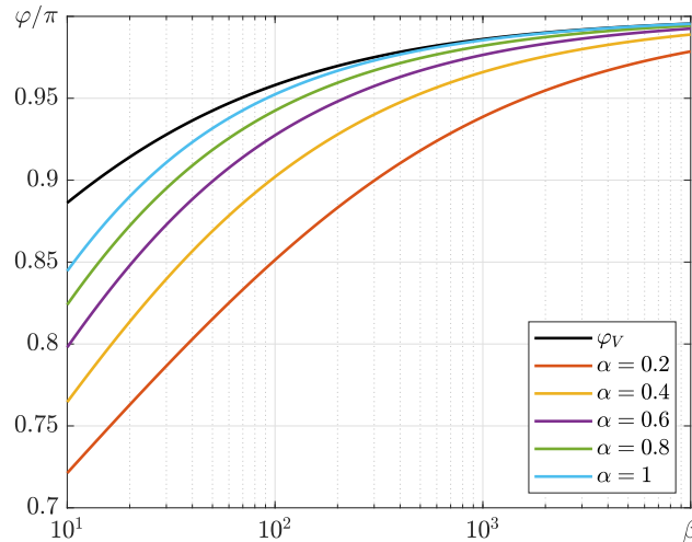
Рис. 2. Зависимость сдвига фаз поступательных \varphi_V (чёрная линия) и вращательных \varphi_\Omega (цветные линии) колебаний корпуса от \beta
