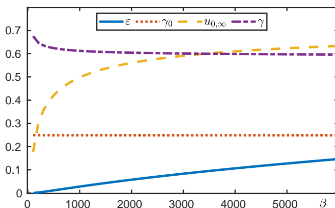
Рис. 5. Эффективность движения ( \varepsilon ), скорость ( u_{0,\infty} ), соотношение масс ВР ( \gamma ) и амплитуда колебаний ВМ ( \gamma_0 ) при \Theta_0 = 1.3 , \phi = 0.85
