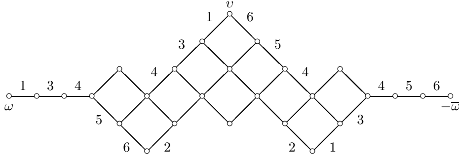
Рис. 1. (E_6, \varpi_1) .
