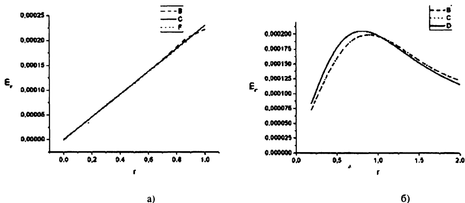
Рис.3. Напряженности собственного электрического поля E_r для равномерного и гауссовского распределения плотности заряда пучка.
