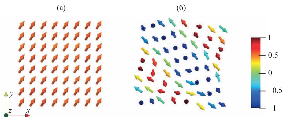
Рис. 1. Основные состояния спиновой модели Гейзенберга на квадратной решетке ( J = 1 ), возникающие при T \rightarrow 0 : (а) без взаимодействия Дзялошинского – Мории, (б) с учетом взаимодействия Дзялошинского – Мории. Размер системы N = 64 . Каждый спин представлен стрелкой. Цвет стрелок представляет собой функцию координаты z между направлением спина вниз -1 (синий) и вверх +1 (красный)
