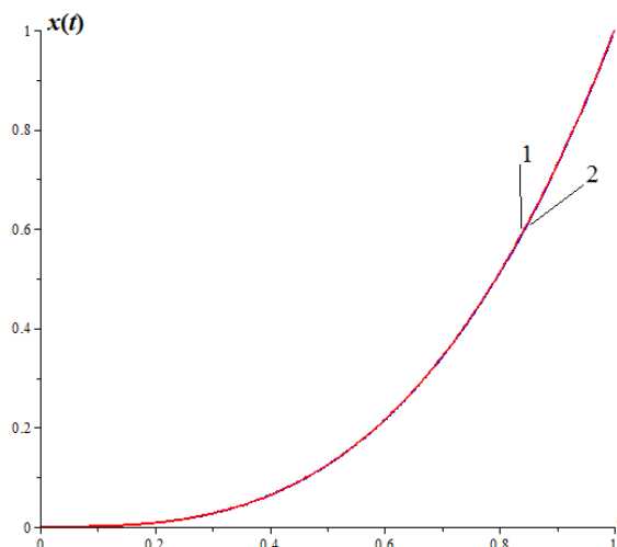
Рис. 1. Конечно-разностная явная схема (кривая 1) и точное решение (кривая 2)
